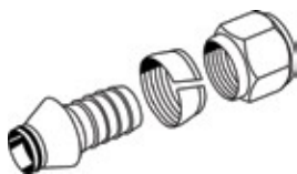
Концовка разборная 3/4" (евроконус)
